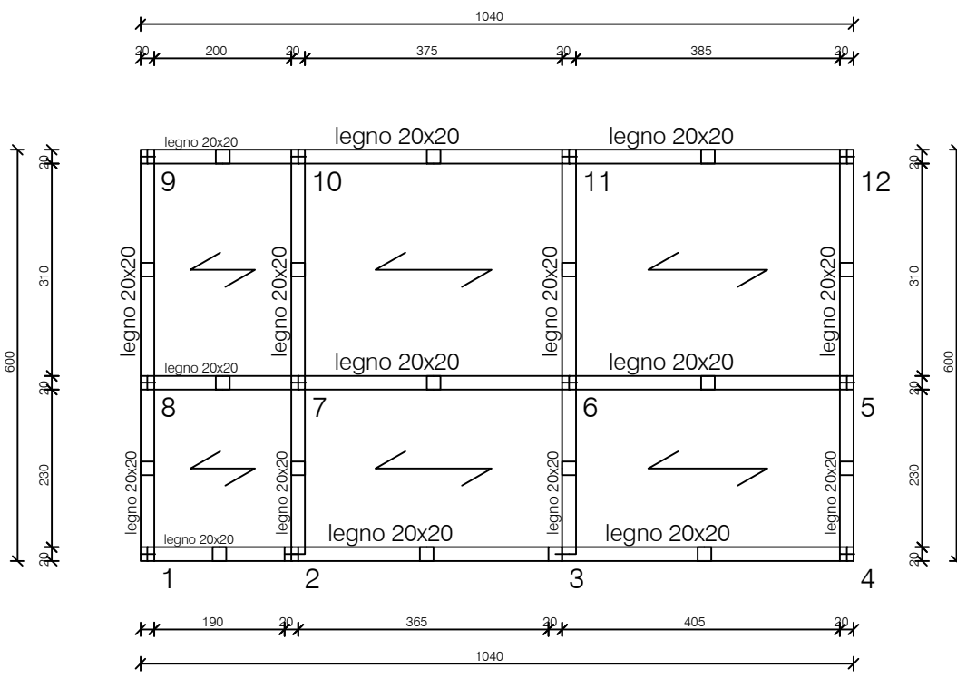
PIANTA IMPALCATO QUOTA m: 3.70
