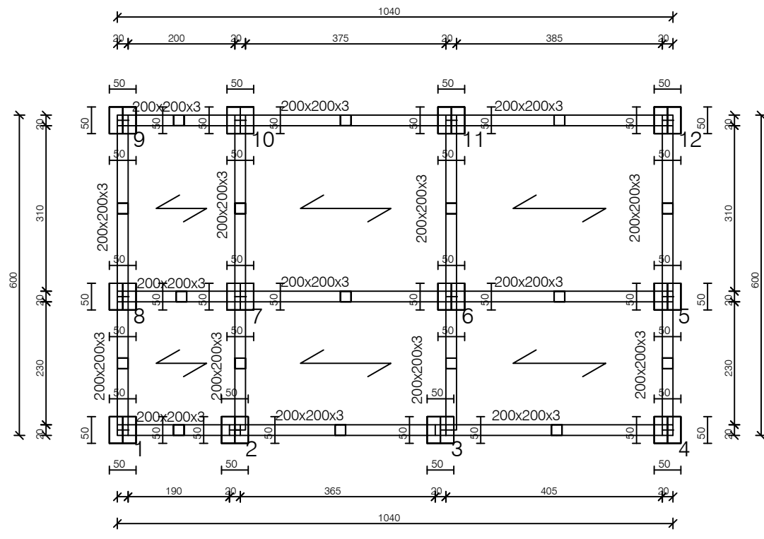
PIANTA IMPALCATO QUOTA m: 0.00
