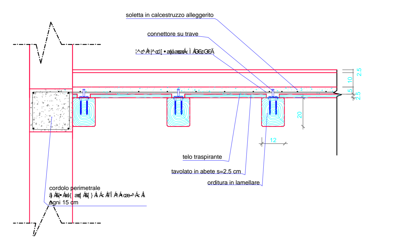
Sezione A-A
