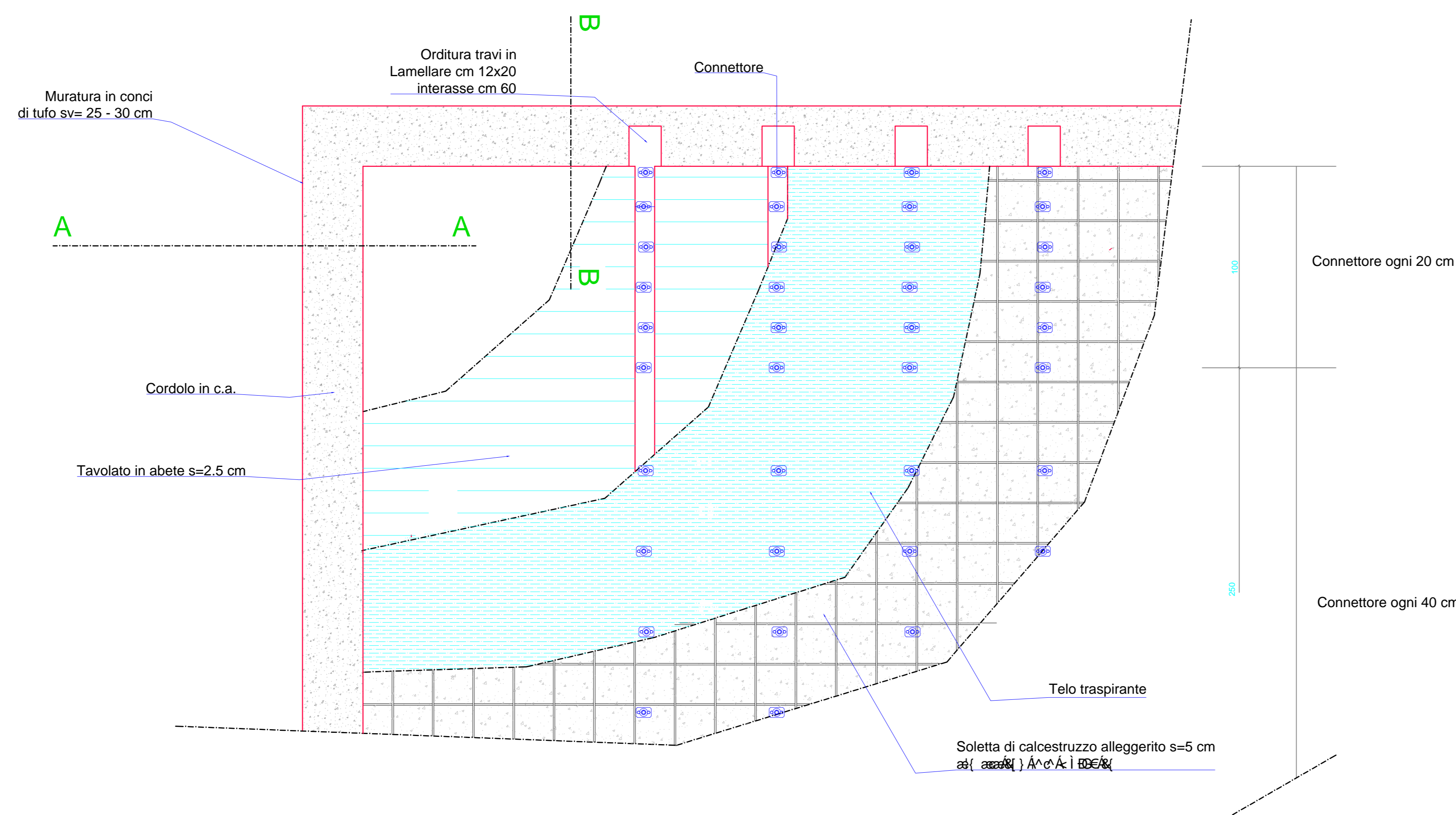
PARTICOLARE COLLEGAMENTO ALLA MURATURA TIPOLOGICA Rapp. Scala 1:20
